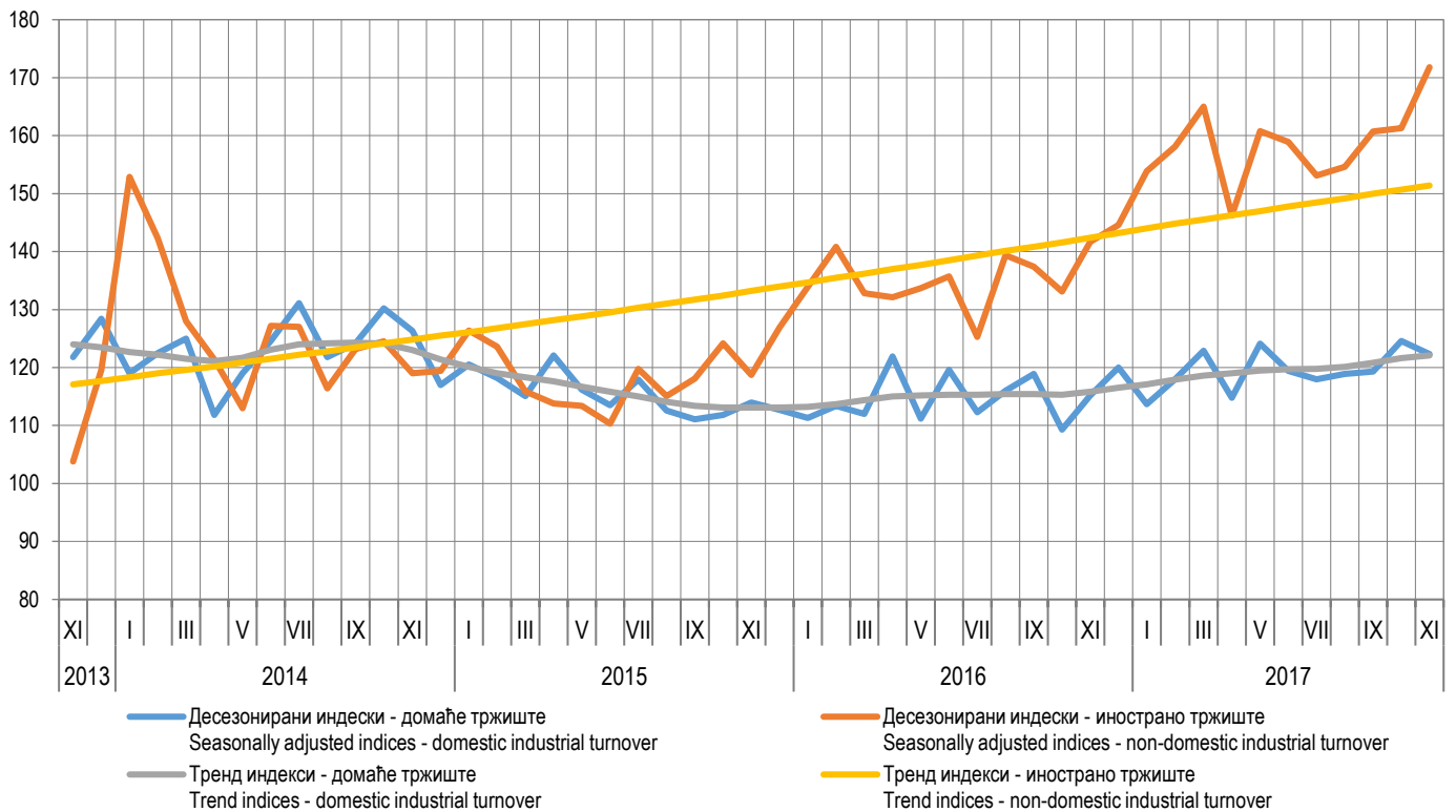
Графикон 1. Индекси промета индустрије, новембар 2013 – новембар 2017. (2010=100) * Graph 1. Industrial turnover indices, November 2013 – November 2017 (2010=100) *
